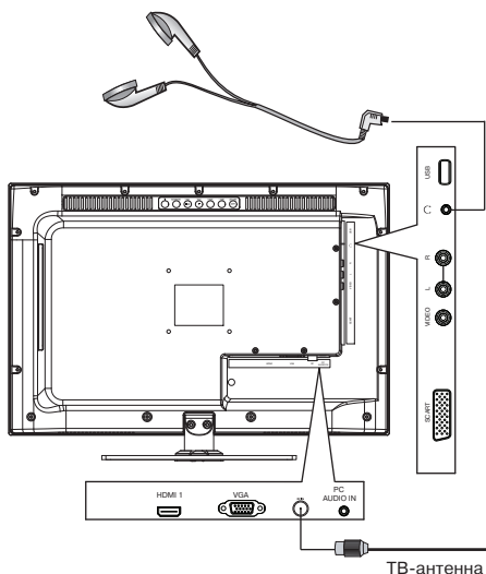
ТВ-антенна
