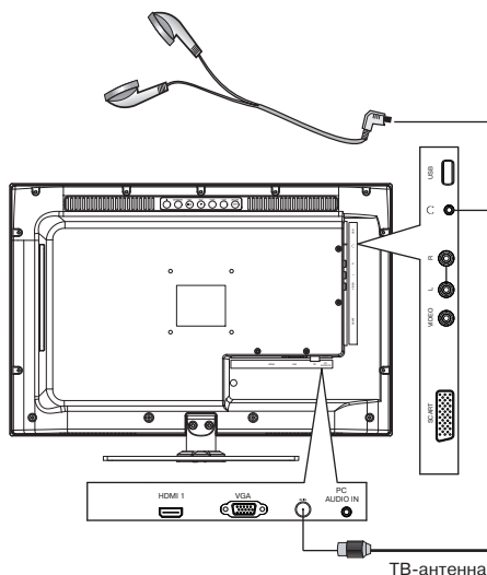
ТВ-антенна
