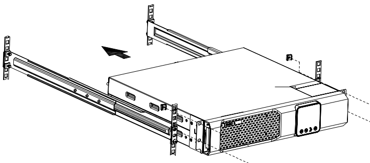
Рис. 5. Установка ИБП (этот же метод используется для батарей)
