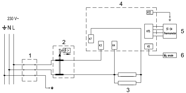
Електросхема
