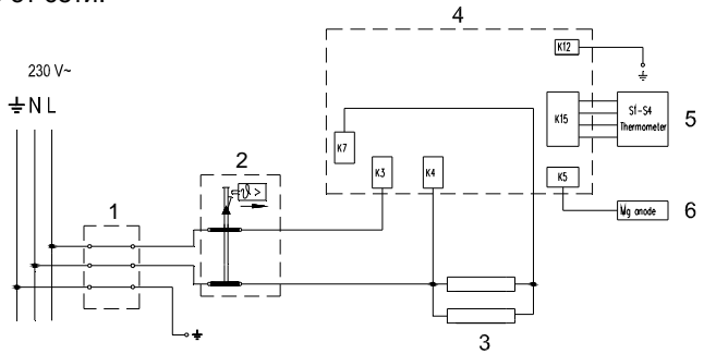
Электросхема
