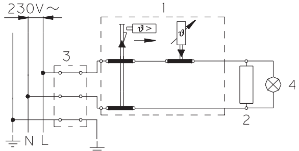
Схема електричного підключення
