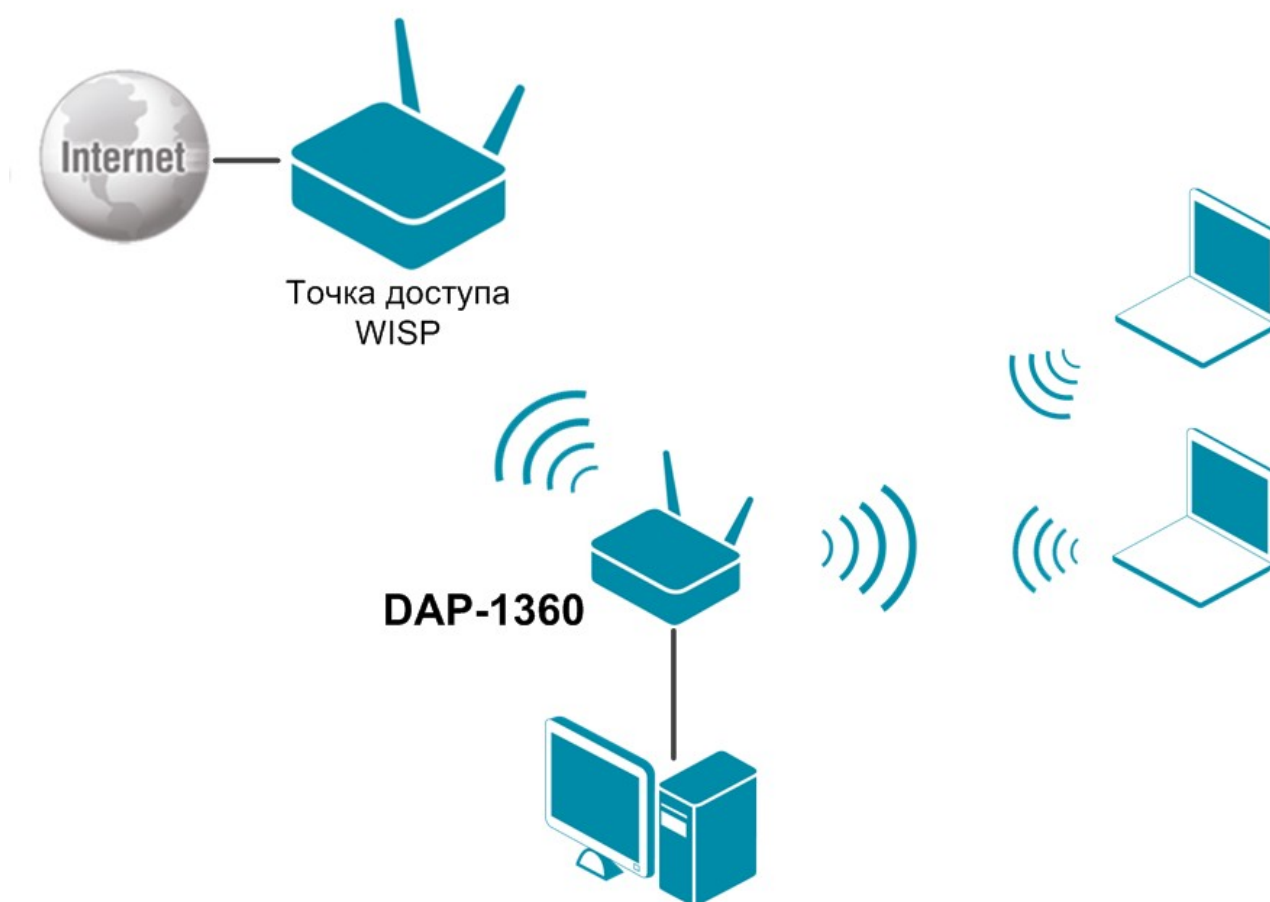
Рисунок 140. Подключение DAP-1360U в режиме маршрутизатора в качестве клиента.
