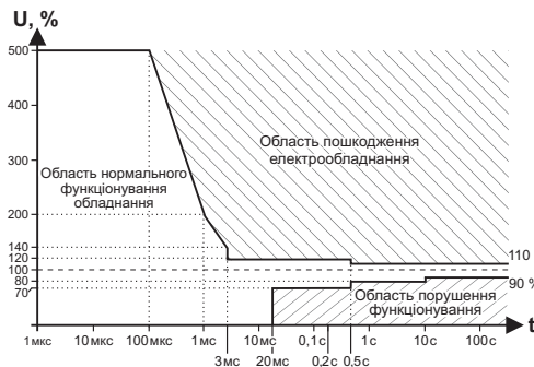
Рис. 1. Крива роботи електрообладнання ITIC (CBEMA), ( http://www.home.agilent.com/upload/cm_upload/All1.pdf?&cc=UA&lc=eng ).
