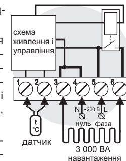
Схема 1. Схема підключення та спрощена внутрішня схема
