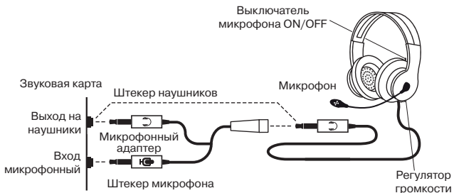
Рис. 1. Схема подключения
