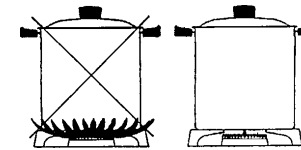
Рис.2 Установка каstrюли на решетке стола
