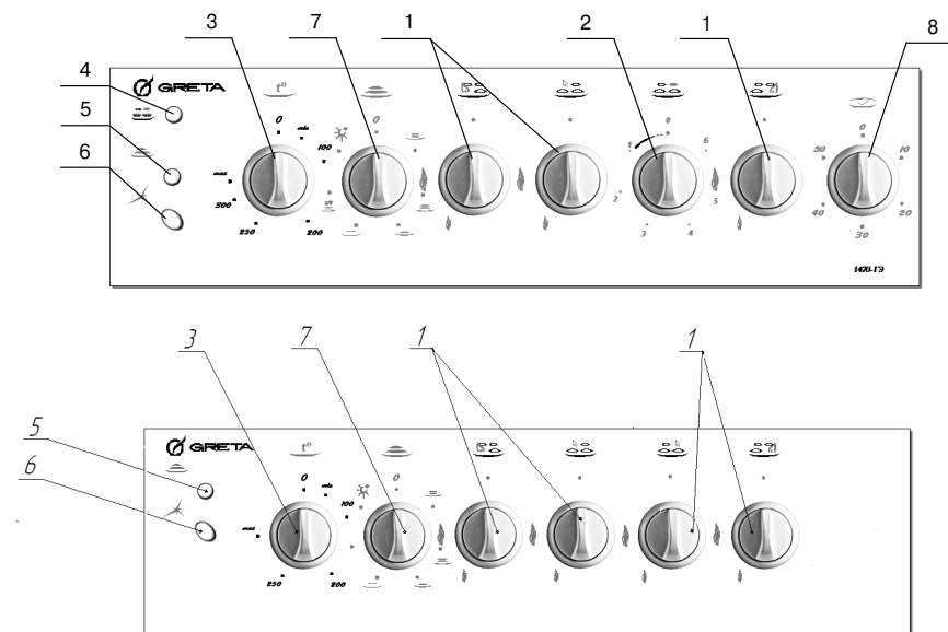
Рис 9 Панель управления
