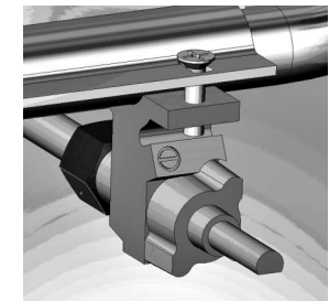
Рис. 6 Кран газовый с винтом малого пламени
