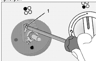
1 Гвинт регулювання подачі газу
