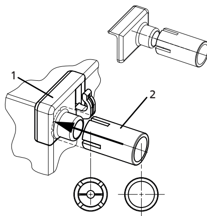
Мал. 1. Надіньте обмежувач (2) на виступ (1) до опору.
