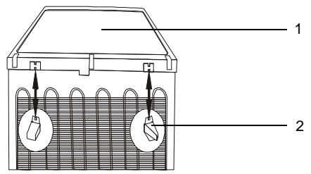
1 - площина установча; 2 - упор. Рисунок Б.2 - Схема кріплення упорів до площини установчої
