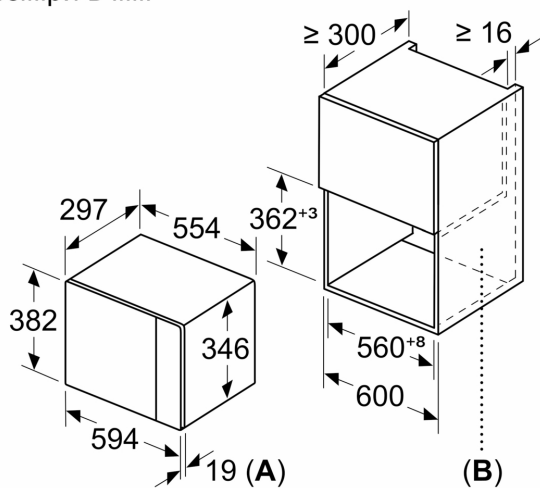
Габарити в мм
