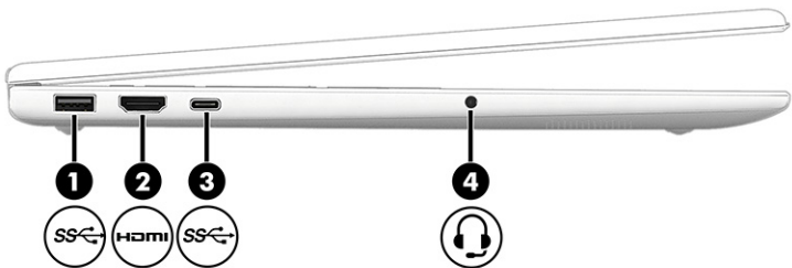
Таблиця 2-2 Компоненти лівої панелі та їх опис
