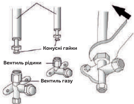
З'єднувальні трубки
