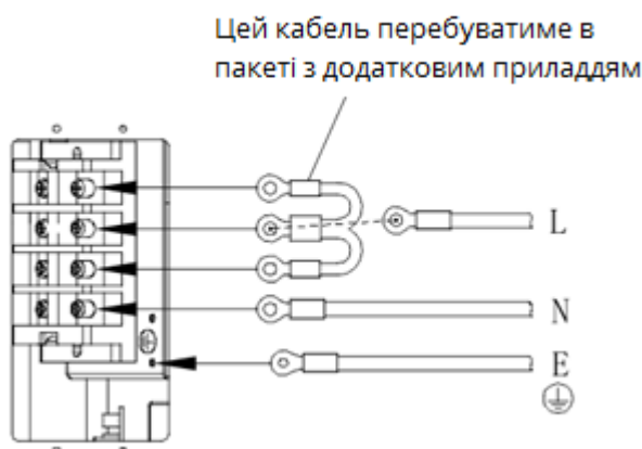
Рисунок 10 Підключення до однофазної електромережі
