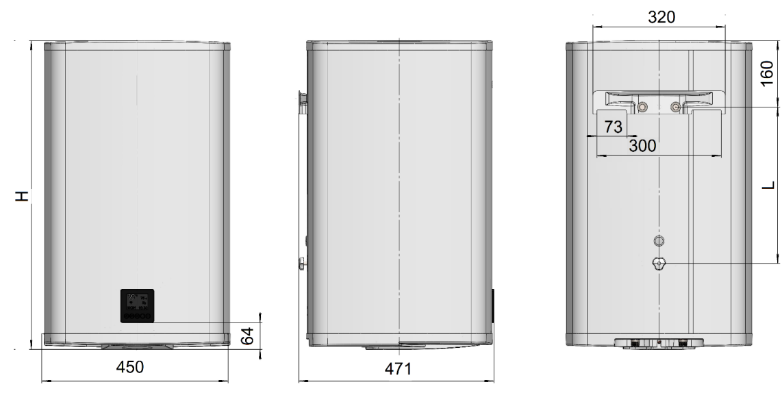
Мал. 3. Монтажні розміри моделей JACK
