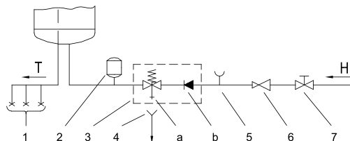
SI. 3: Zatvoreni sistem (pod pritiskom)
