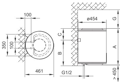
Sl. 1: Vertikalno montiranje na zid
