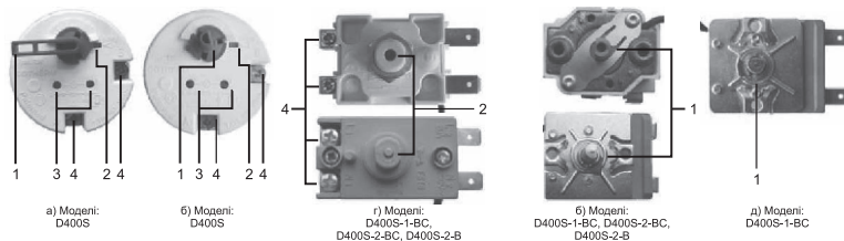
Рисунок 3. Зовнішній вигляд терморегулятора 1 – Регулятор температури; 2 – Кнопка теплового захисту; 3 – Гнізда підключення сигнальної лампи; 4 – Клеми підключення до електроенергії
