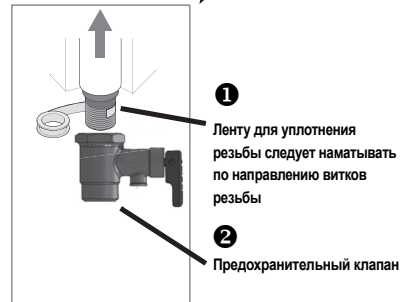
Подсоединение трубопровода с холодной водой
