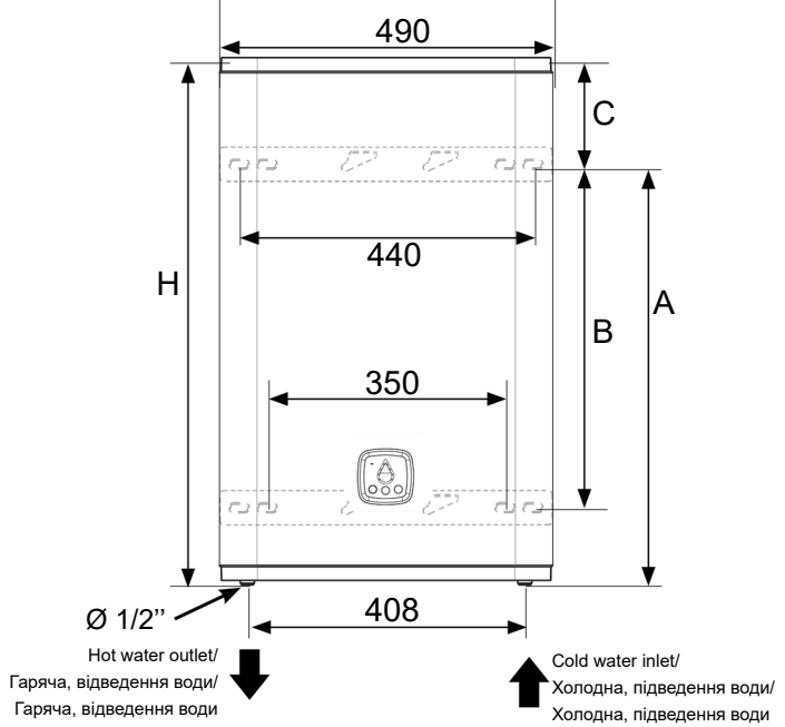
Horizontal wall-mounted/ Горизонтальний настінний водонагрівач/ Горизонтальний настінний водонагрівач
