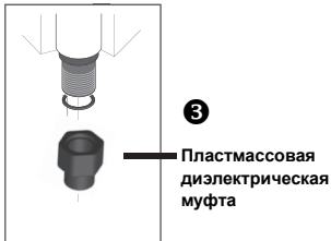
Подсоединение трубопровода с горячей водой
