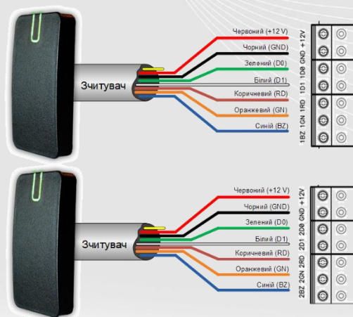
Рис.10. Підключення зчитувачів
