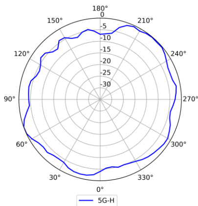
5G (Horizontal)
