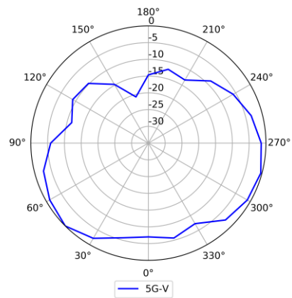
5G (Vertical)
