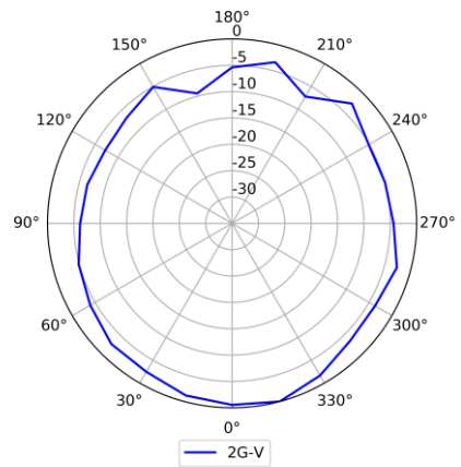
2.4G (Vertical)
