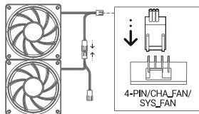
Connect Fan
