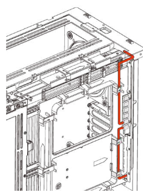
5 Fan cable channel
