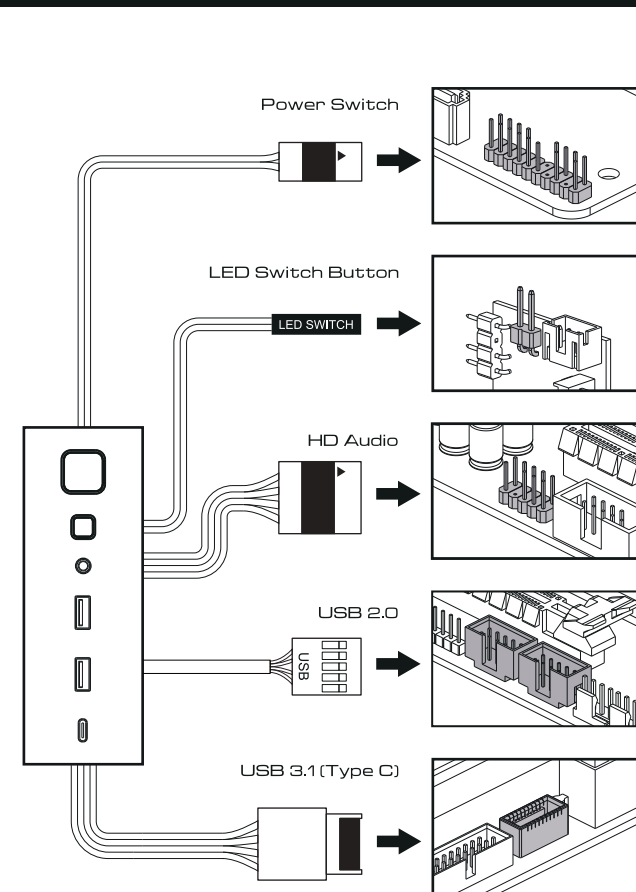
▼ I/O cables
