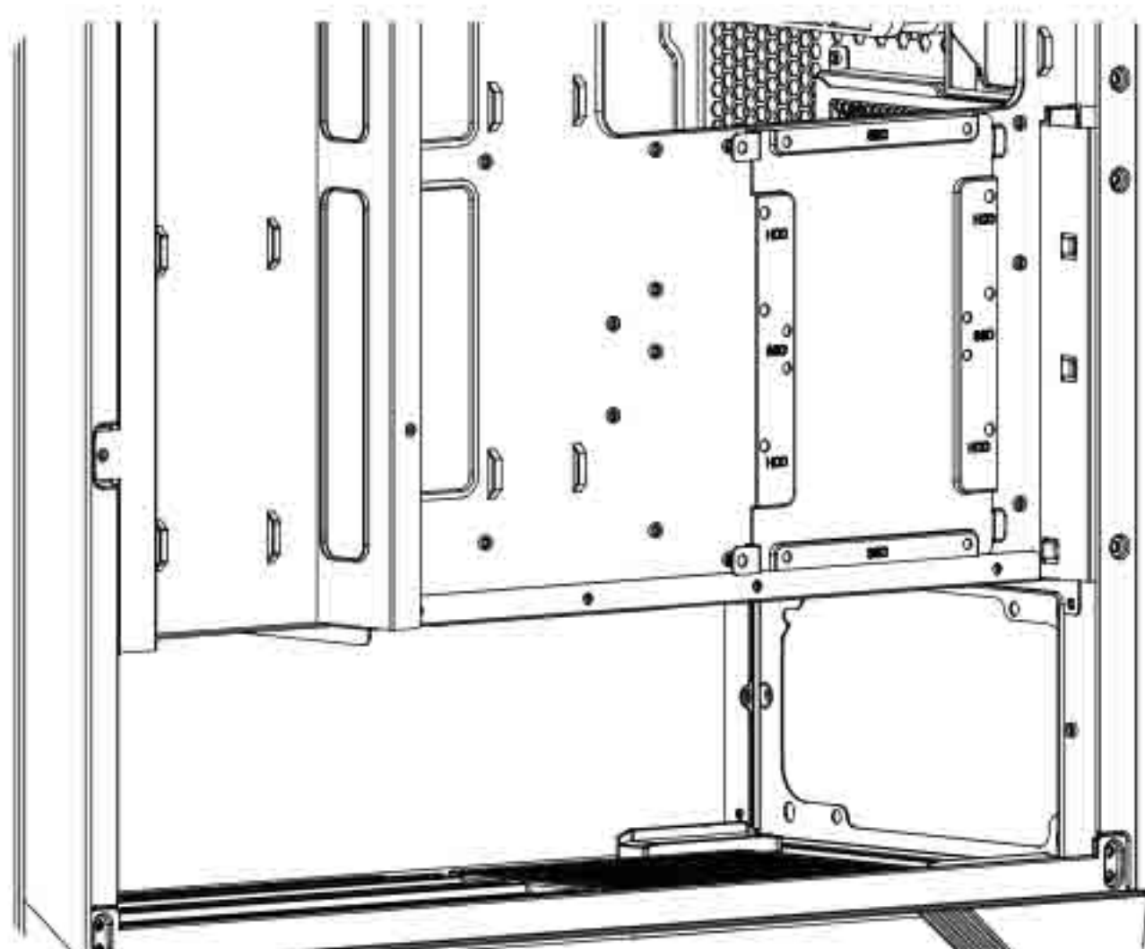
PSU LOCATION LOKALIZACJA ZASILACZA
