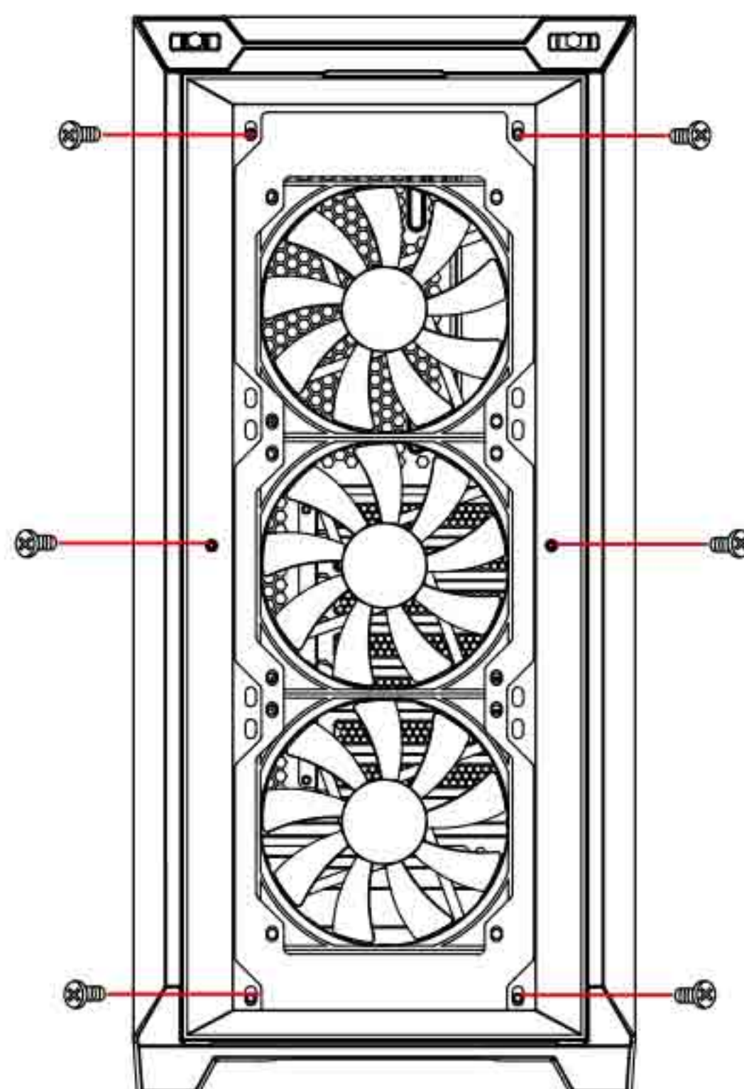
INSTALL 120 MM FANS AND FIX THEM WITH SCREWS ZAŁÓŻ WENTYLATORY 120 MM I PRZYMOCUJ ŚRUBAMI
