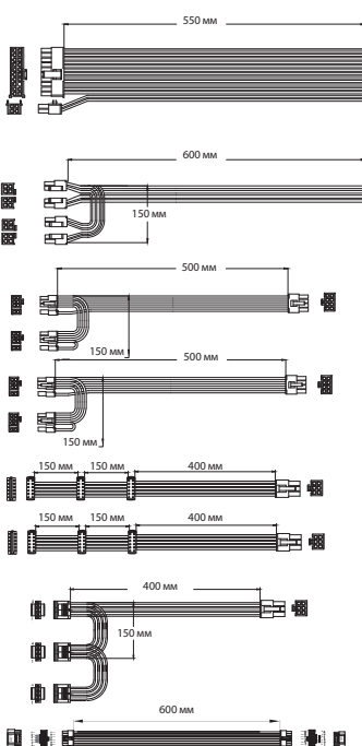
Розніми живлення материнської плати
