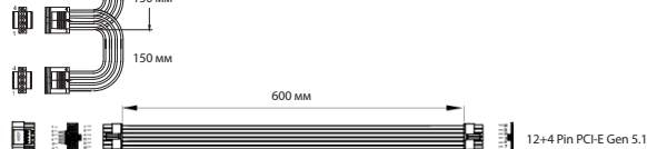
12+4 Pin PCI-E Gen 5.1
