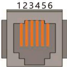
Роз'єм RJ11
