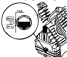
Рисунок 2. Схема перевірки рівня мастила в картері компресора.
