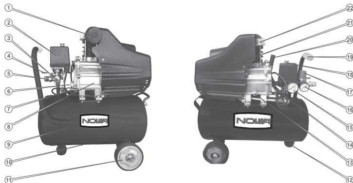
Рисунок 1. Загальний вигляд компресорів моделей «KBN 220-24», «KBN 220-50».
