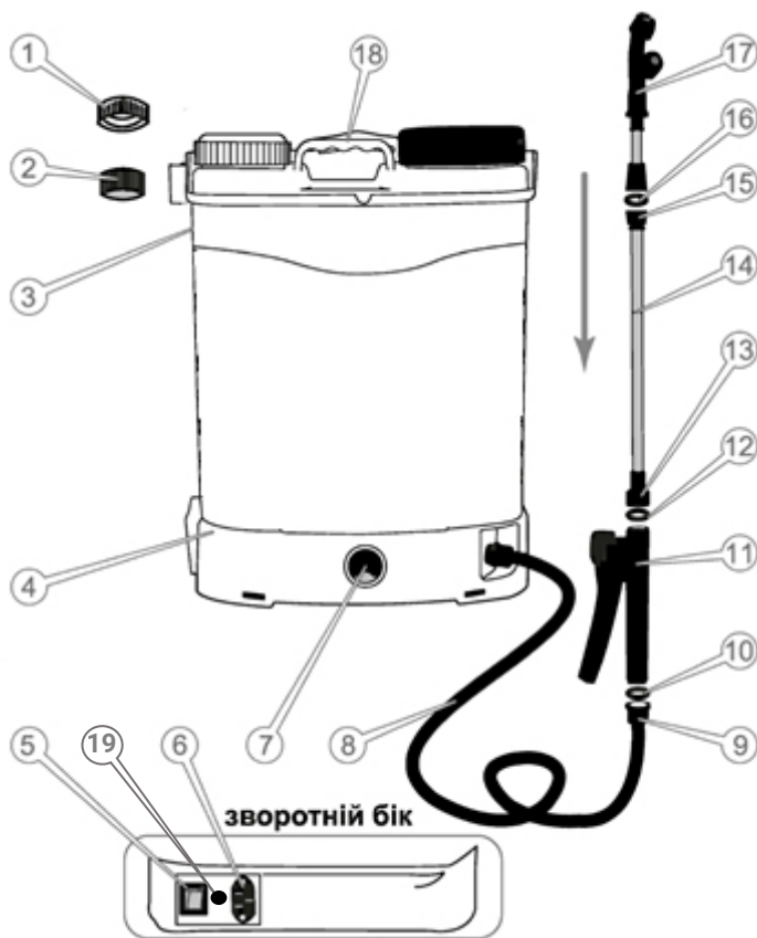
Рисунок 1. Загальний вигляд обпрыскавача акумуляторного ТМ «NOWA», моделей «OP 1810k» та «OP 1812k».
