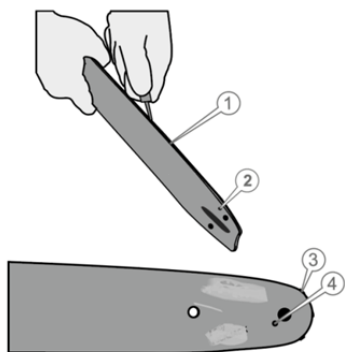
Рисунок 9. Схема обслуговування «шини»
