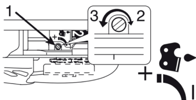
Рисунок 4. Регулювання обсягу автоматичної подачі мастила на ланцюг.
