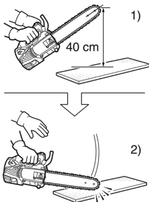
Рисунок 6. Схема перевірки роботи інерційного гальма ланцюга.
