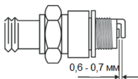
Рисунок 15. Свічка запалювання. Рекомендований зазор між електродами.
