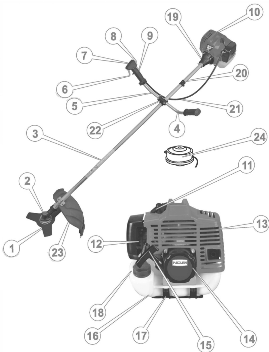
Рисунок 1. Загальний вигляд мотокози ТМ «Vitals», моделі «BK 251n».
