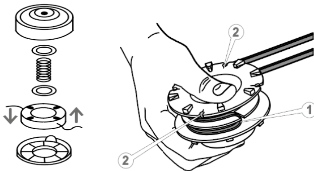
Рисунок 15. Схема заміни жилки у різальній головці.
