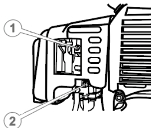
Рисунок 17. Схема розташування гвинтів регулювання карбюратора.
