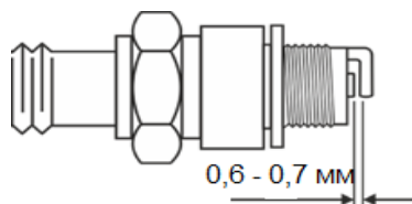
Рисунок 16. Свічка запалювання. Рекомендований зазор між електродами.
