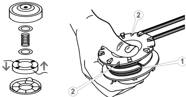
Рисунок 15. Схема заміни жилки у різальній головці.
