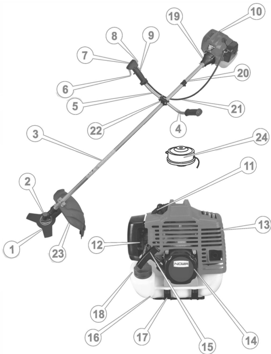
Рисунок 1. Загальний вигляд мотокози ТМ «NOWA», моделі «Professional TB 5240n».
