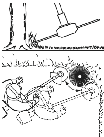
Рисунок 13. Схема скошування трави навколо дерев.
