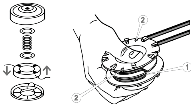
Рисунок 15. Схема заміни жилки у різальній головці.
