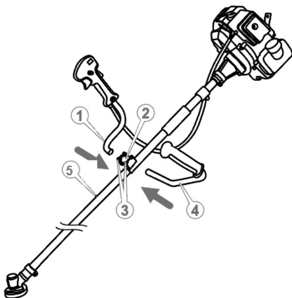
Рисунок 3. Схема встановлення руків'їв виробу.
