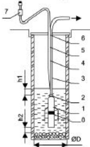
Рис. 3 Встановлення насоса для роботи автономно
