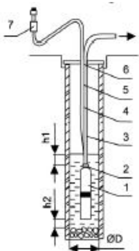
Рис. 3 Встановлення насоса для роботи автономно
