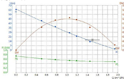
3QGD-750
