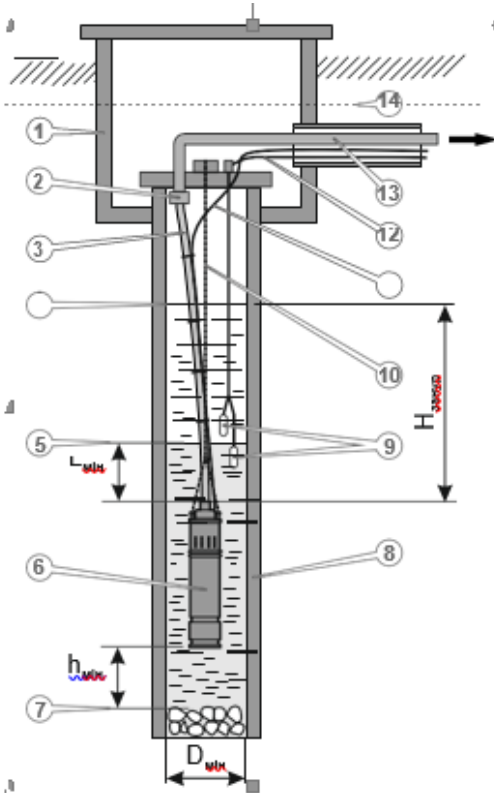
Рис. 2 Встановлення насоса для роботи у стаціонарних умовах
