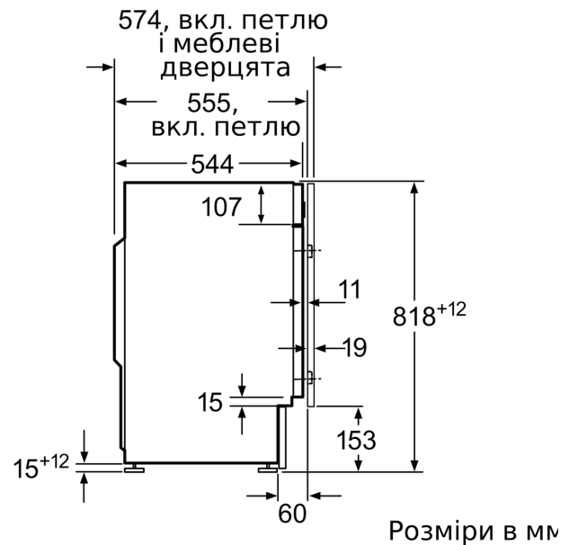
Деталь Z
