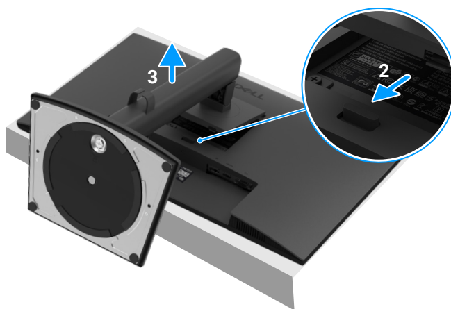
Зображення 19. Витягніть підставку з монітора
