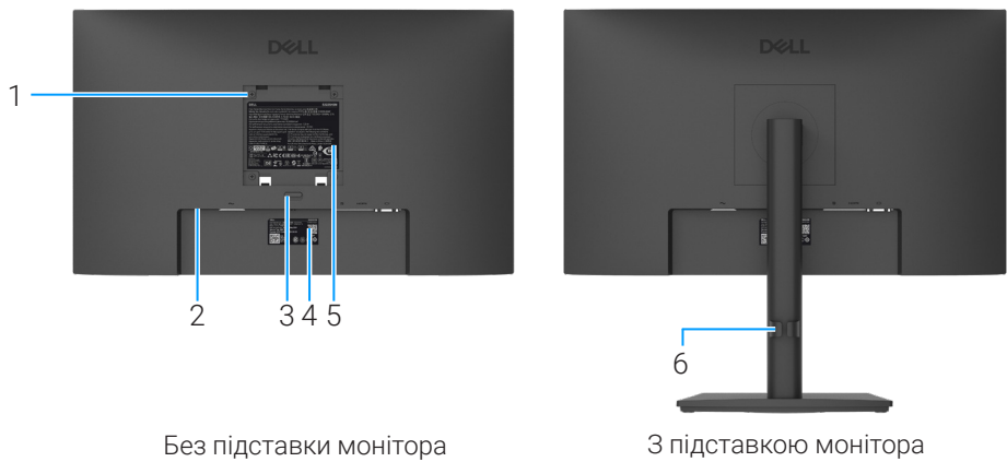
Зображення 2. Вид ззаду
