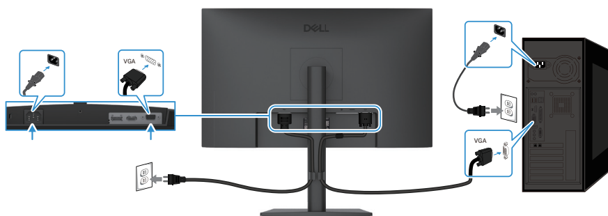
Зображення 14. Підключення кабелю VGA
